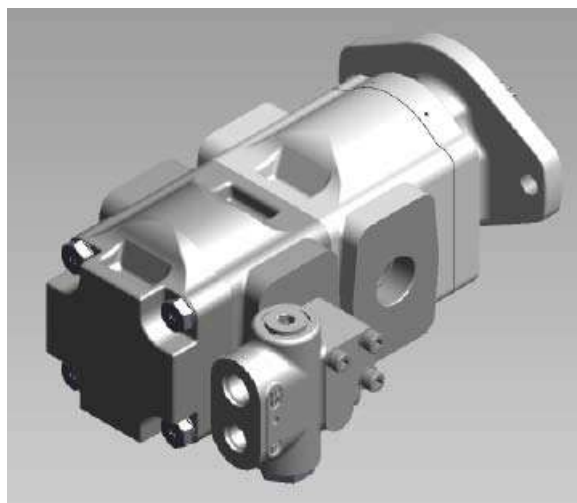
Vanne prioritaire à détection de charge avec signal de sensibilité à la charge dynamique Fonction « F »
