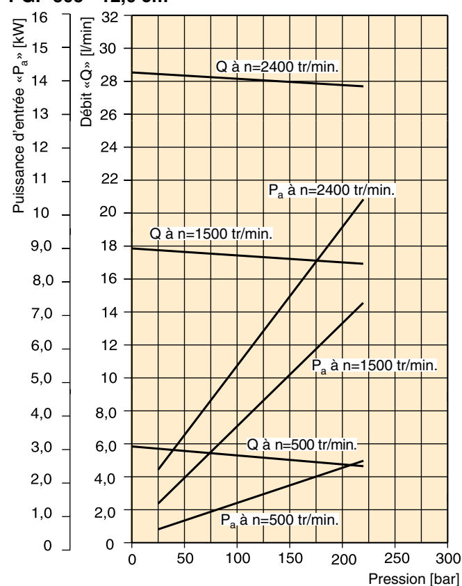
PGP 505 - 12,0 cm 3
