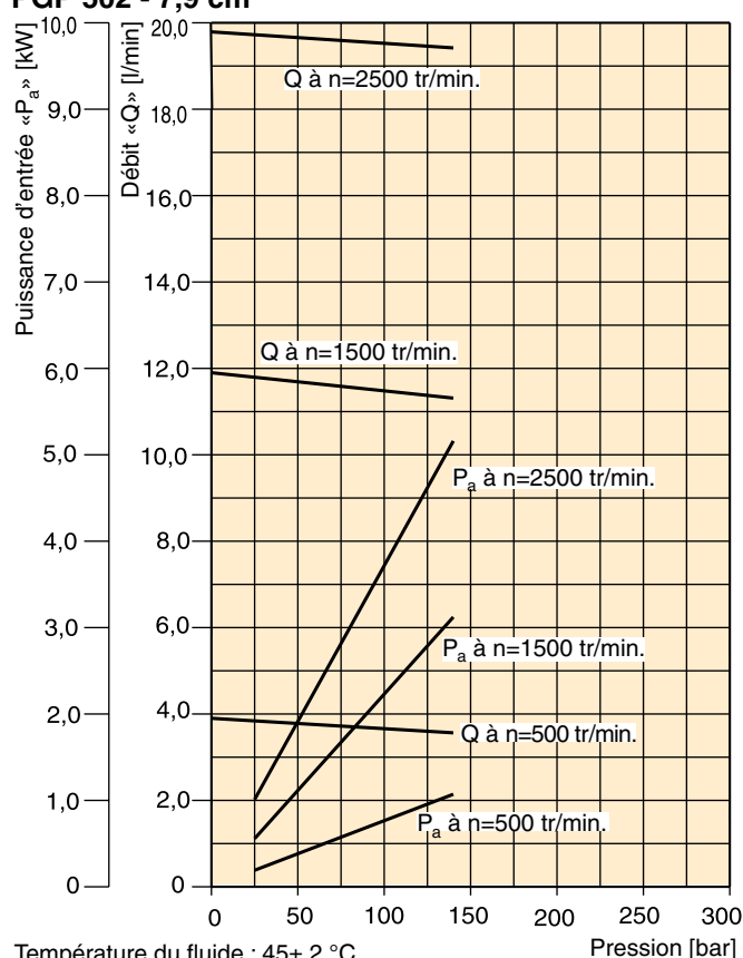
PGP 502 - 7,9 cm 3
