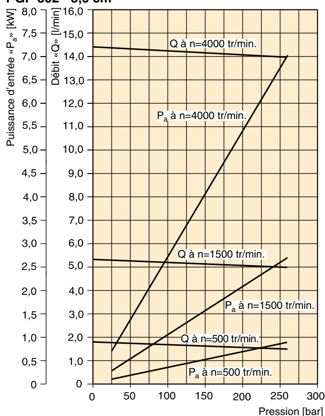
PGP 502 - 3,6 cm 3
