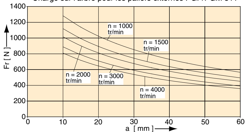
Charge sur l'arbre pour les paliers externes PGP/PGM 511
