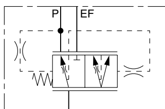
Diviseur de débit Fonction « A »
