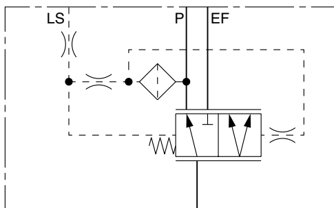
Vanne prioritaire à détection de charge avec signal de sensibilité à la charge dynamique
