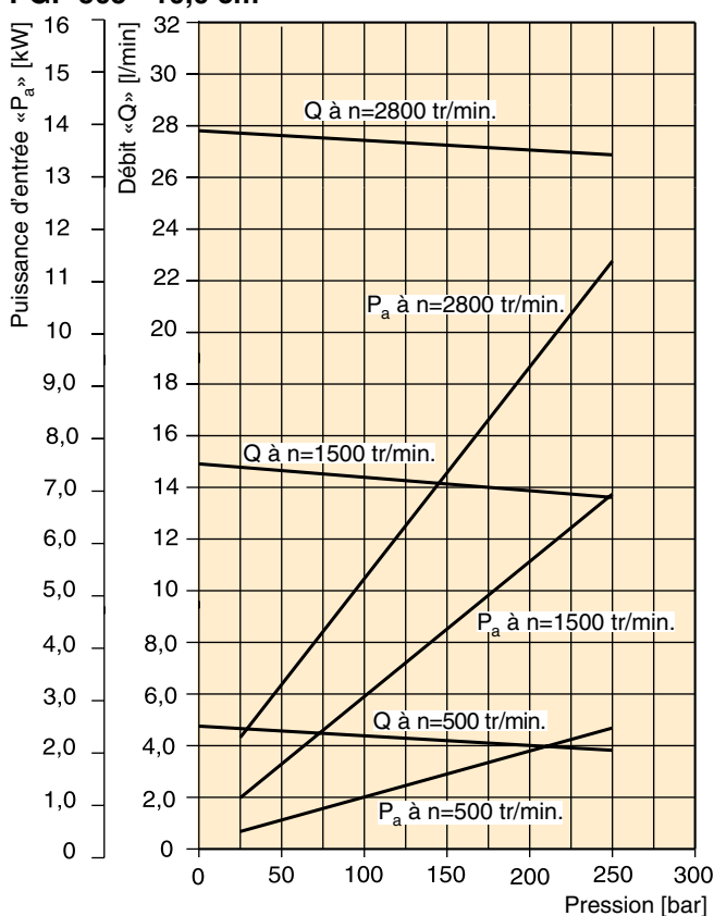
PGP 505 - 10,0 cm 3
