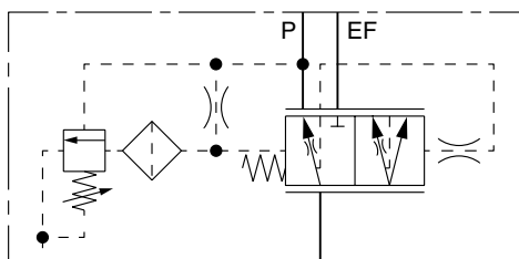
Diviseur de débit avec limiteur pilote Fonction « C »
