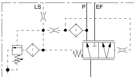
Vanne prioritaire à détection de charge avec signal de sensibilité à la charge dynamique
