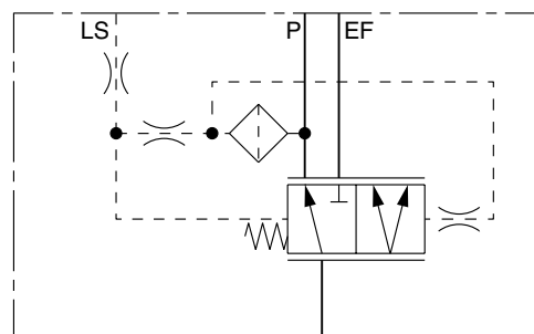
Vanne prioritaire à détection de charge avec signal de sensibilité à la charge dynamique Fonction « F »
