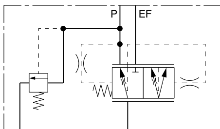
Diviseur de débit avec limiteur plein débit Fonction « B »
