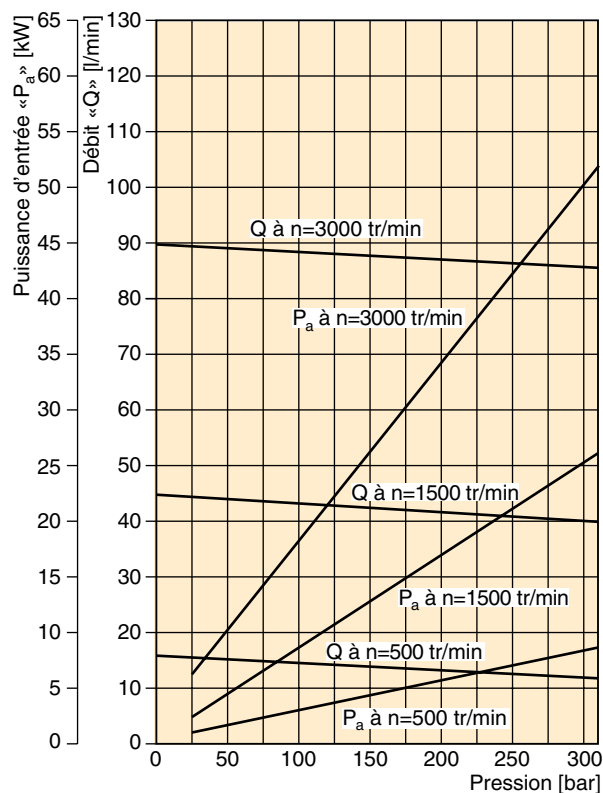
PGP640 - 30,0 cm 3
