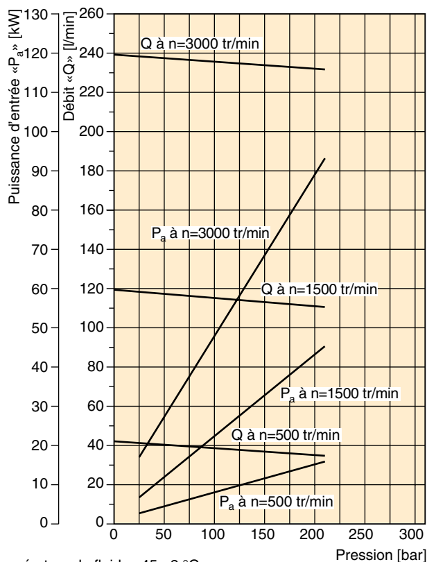
PGP640 - 80,0 cm 3
